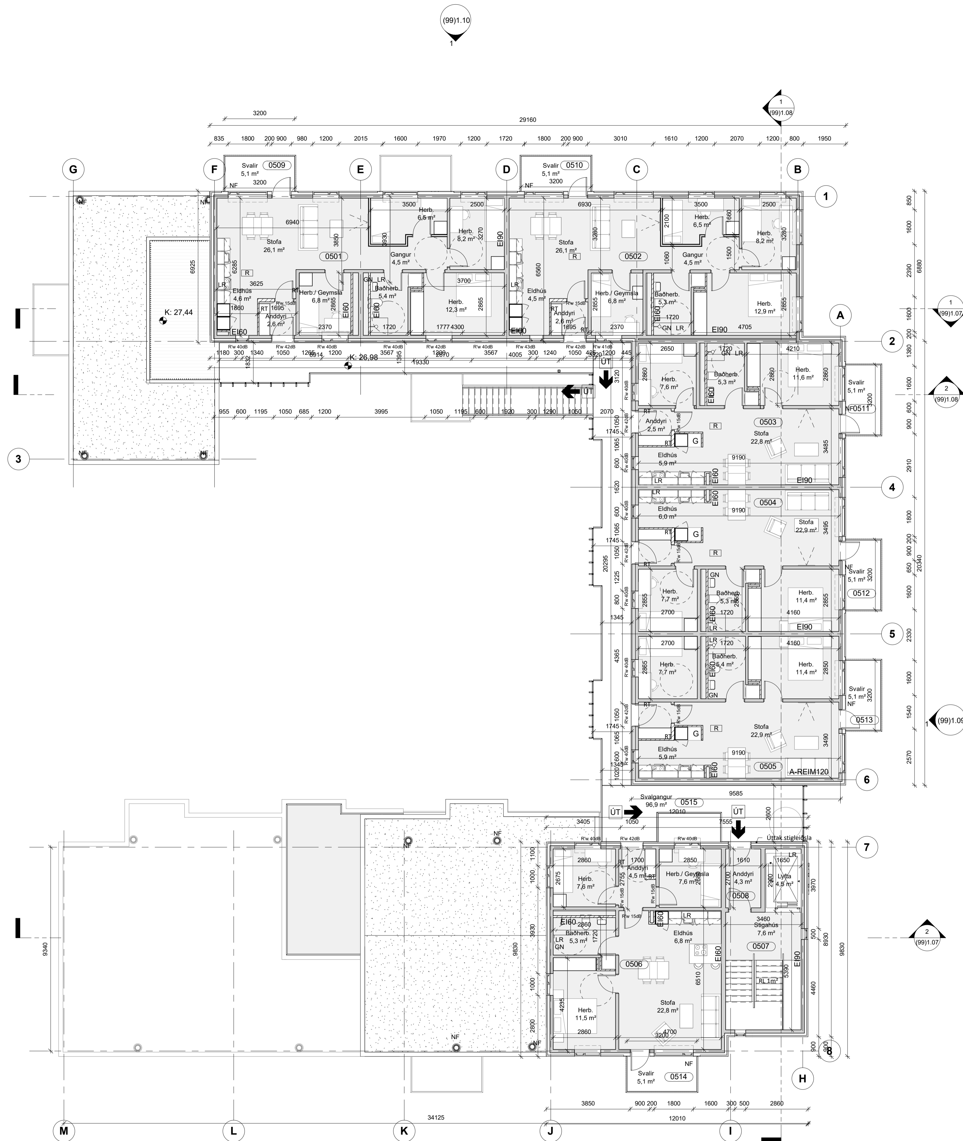
2 Grunnmynd, 5. hæð 1 : 100
