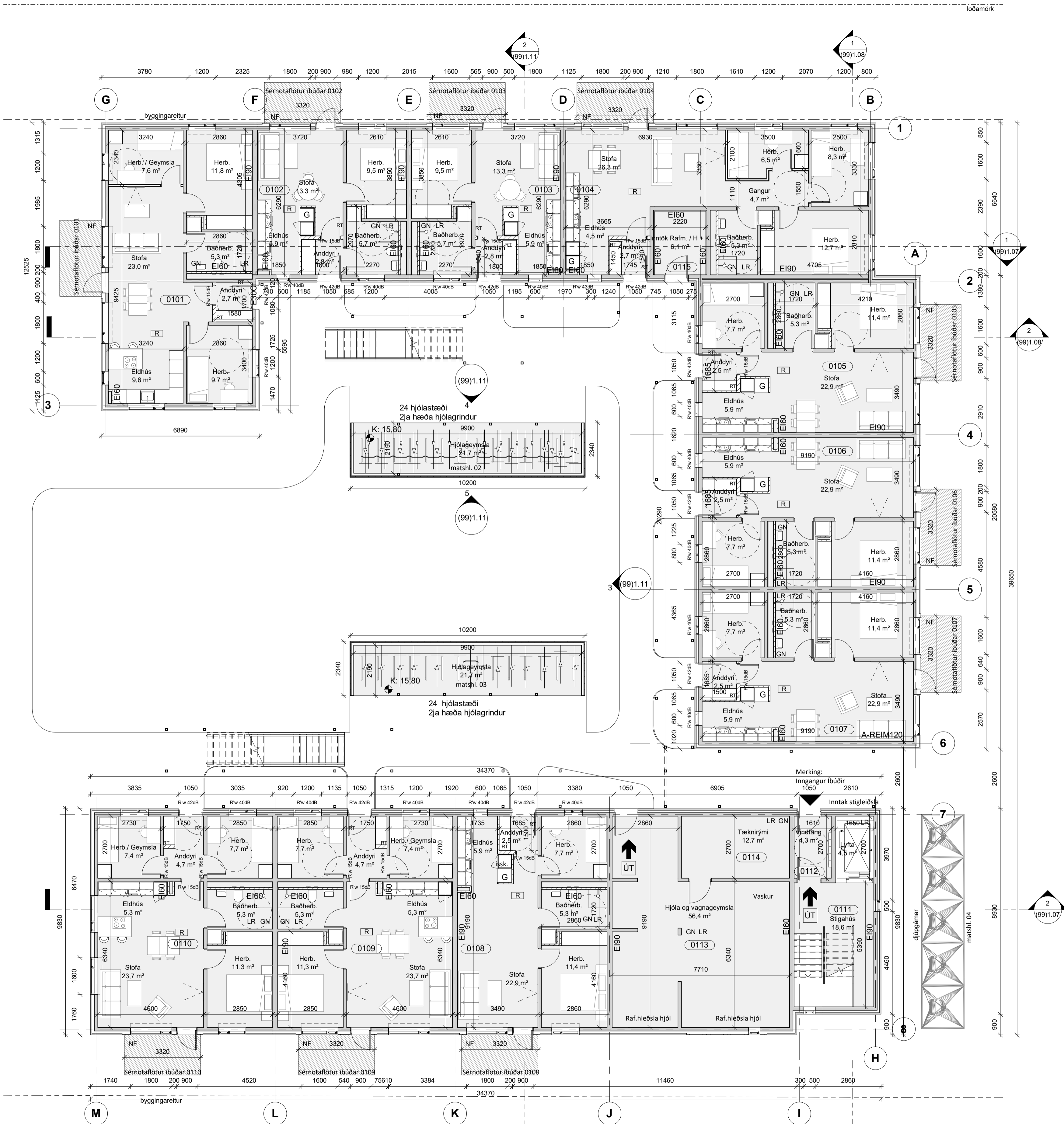
1 Grunnmynd, 1. hæð 1 : 100
